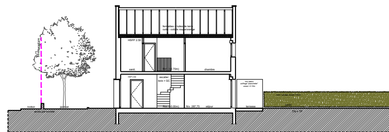
Coupe sur le terrain
