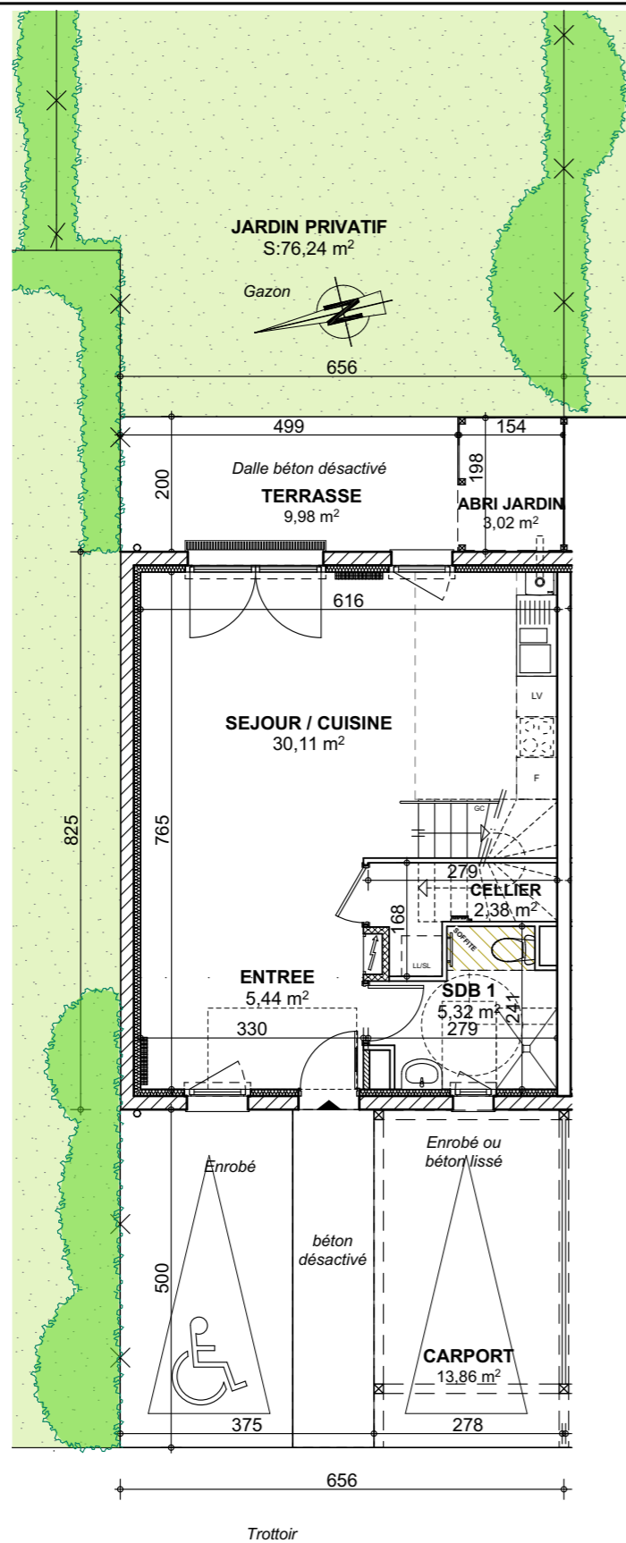
REZ-DE-CHAUSSEE
