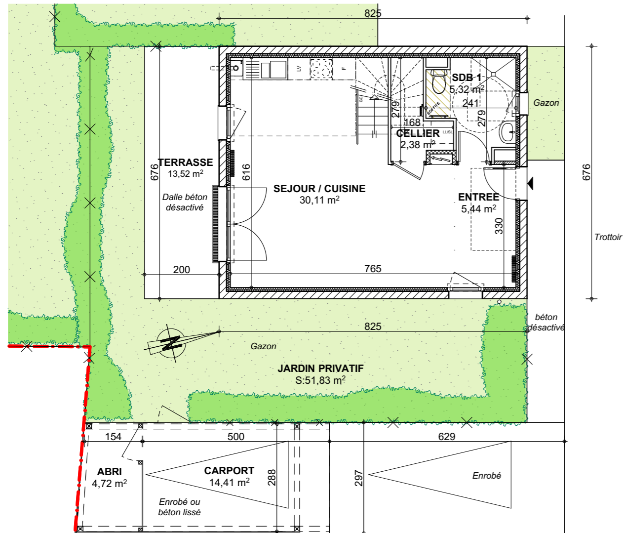
REZ-DE-CHAUSSEE
