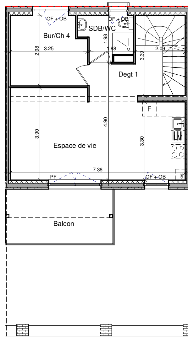
2 R+1 - 05 1 : 100
