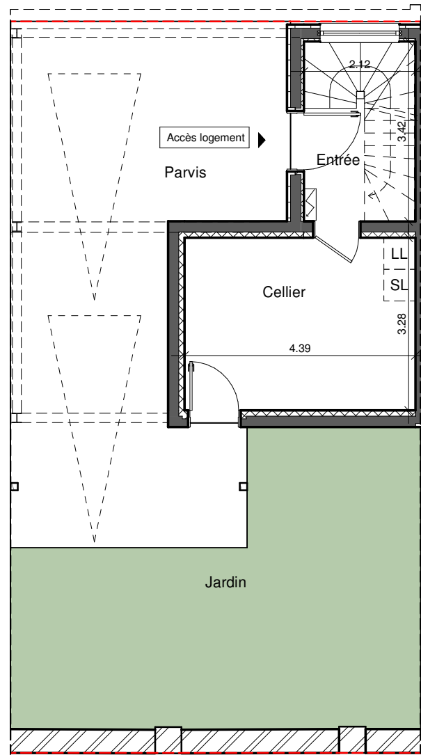
1 RDC - 05 1 : 100
