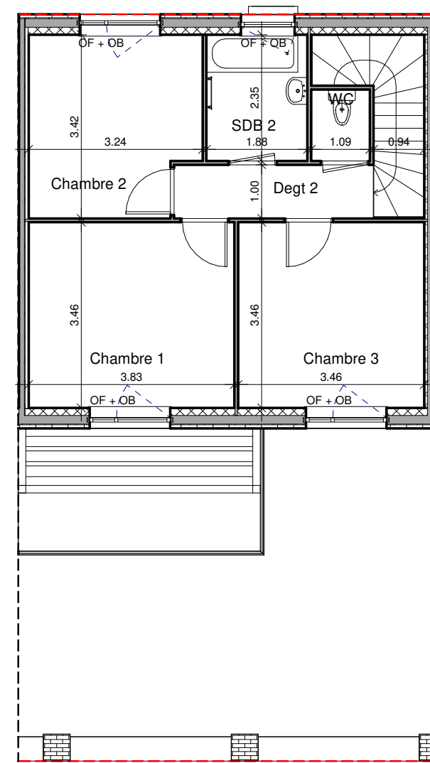
3 Combles - 05 1 : 100
