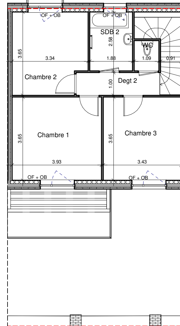
3 Combles - 03 1 : 100
