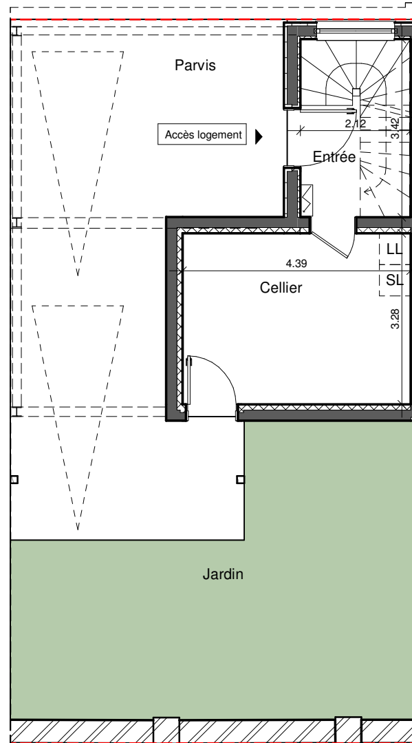
1 RDC - 03 1 : 100
