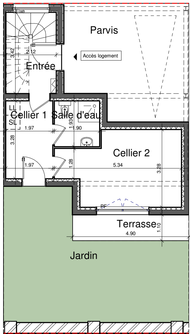
1 RDC - 02 1 : 100
