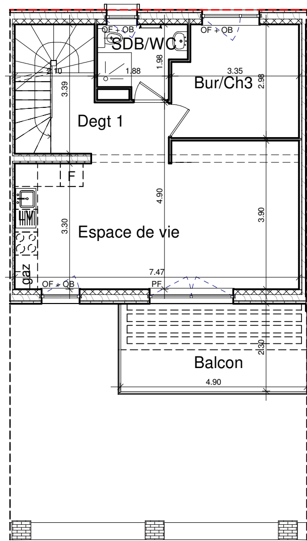
2 R+1 - 02 1 : 100
