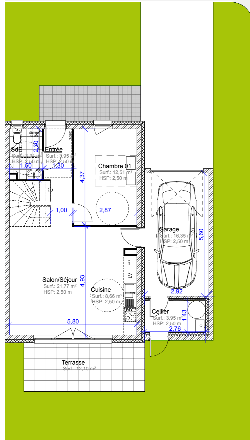
Plan Rez-de-Chaussée
